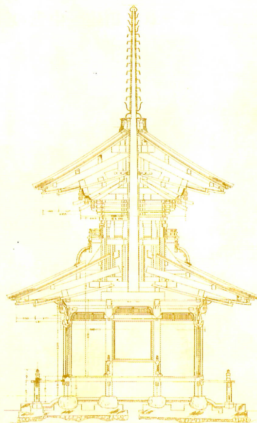
重要文化財 浄妙寺多宝塔 断面図
